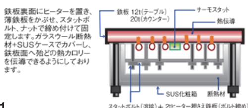
【ヒーター鉄板の断面構造としくみ】
