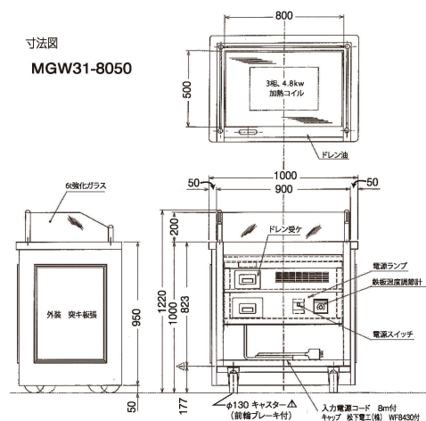
●鉄板寸法図
