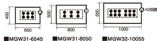
●鉄板寸法図
