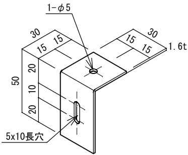
固定金具 4 個付
