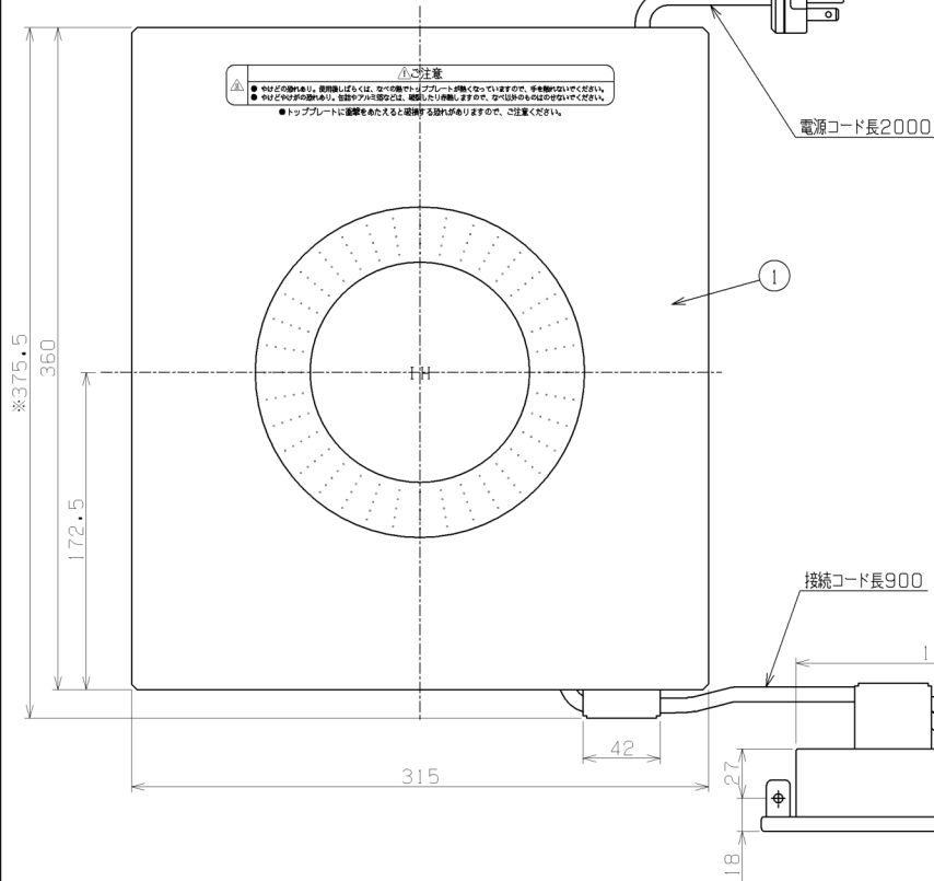
正面図
