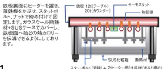
【ヒーター鉄板の断面構造としくみ】
